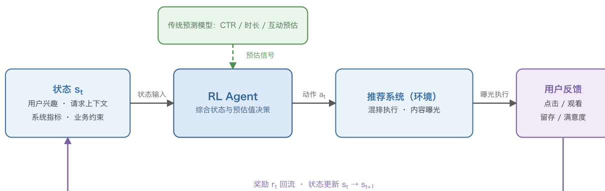
图 28.8: 工业级 RL 推荐系统的闭环框架。
