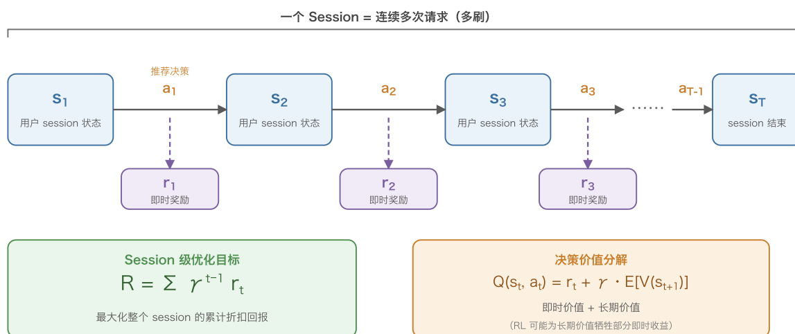
图 28.4: Session 级推荐优化的序列决策建模。
