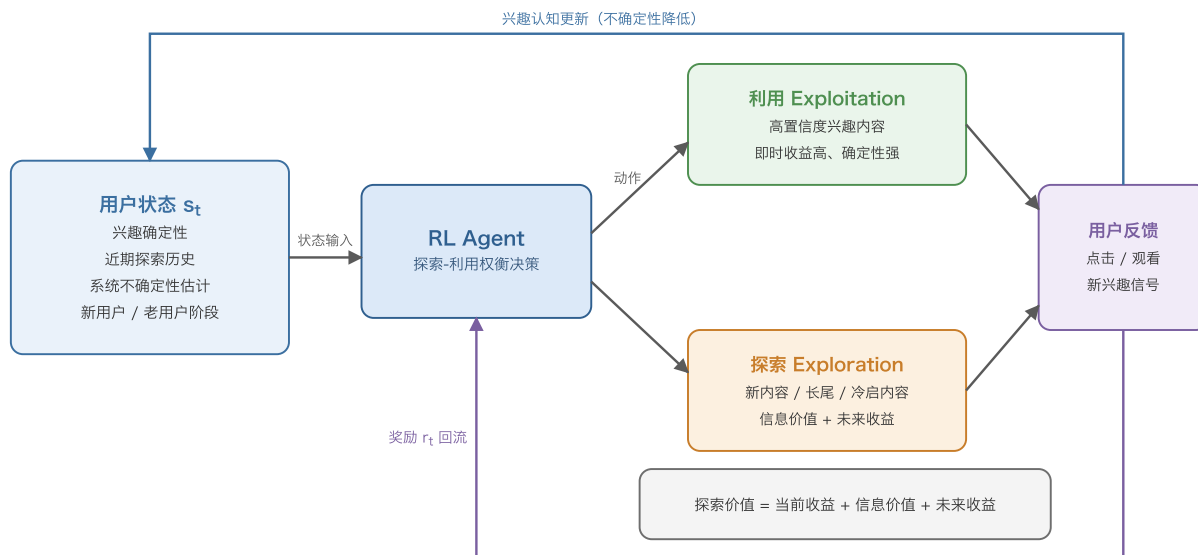
图 28.7: 个性化探索中探索与利用的闭环权衡。
