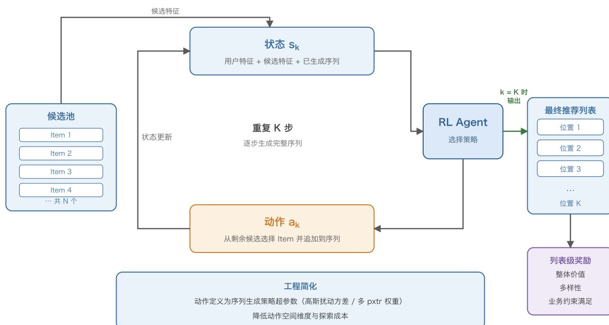
图 28.6: 强化学习序列生成的逐步决策过程。
