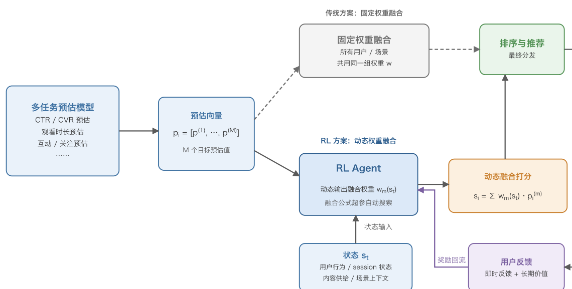
图 28.3: 固定权重融合与 RL 动态权重融合对比。
