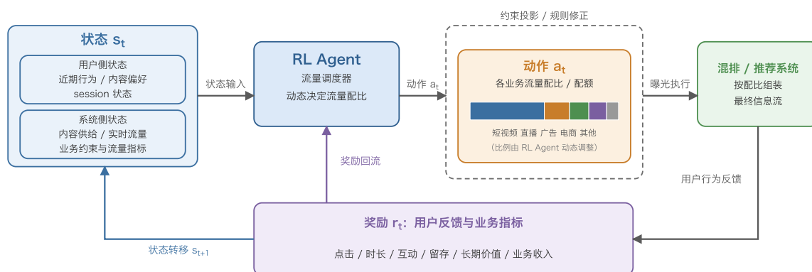
图 28.1: 基于强化学习的流量分配与调控闭环。
