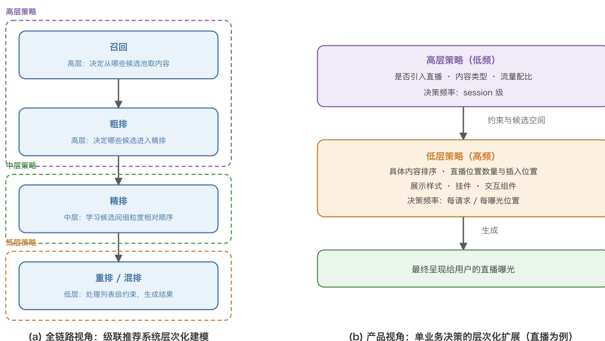
图 28.5: 层次化决策的两种视角。
