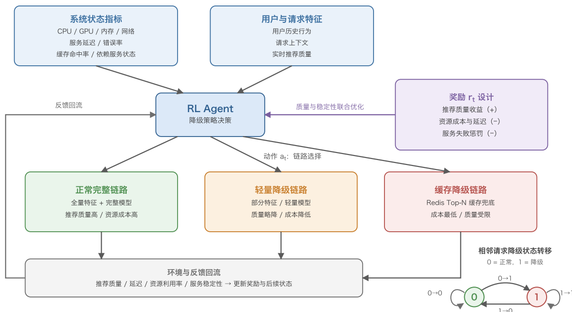
图 28.2: 基于强化学习的流量降级决策（右下角为相邻请求降级状态转移）。
